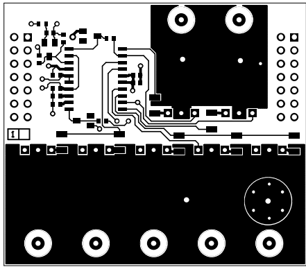
Top Layer 1/2
