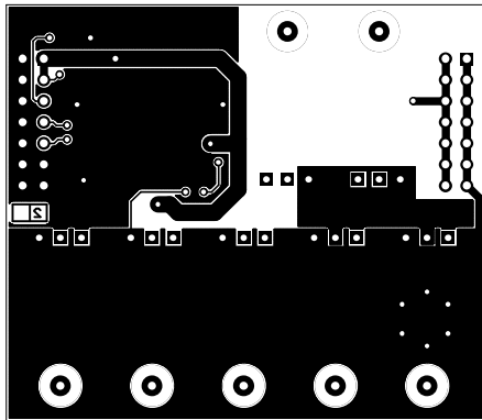
Bottom Layer 2/2
