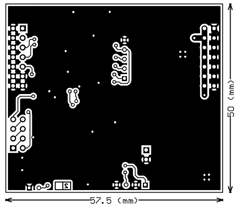
Bottom Layer 2/2
