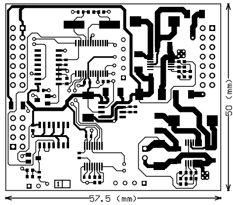
Top Layer 1/2
