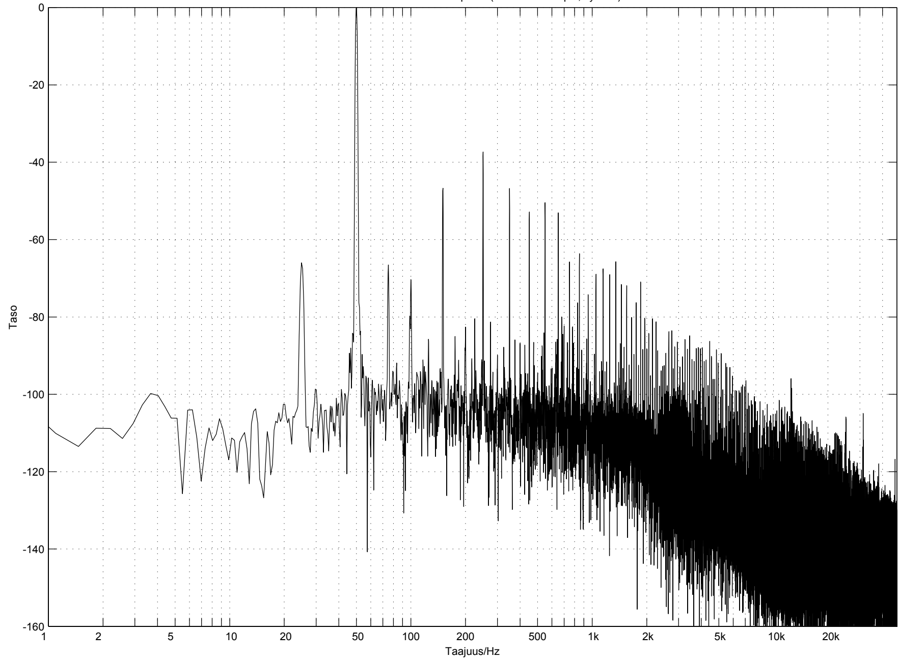
Verkkosähkön normalisoitu spektri (23.8.2003 Kuopio, Jynkkä)
